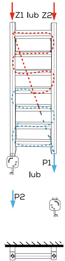
WODNO-ELEKTRYCZNY PODŁĄCZENIE KRZYŻOWE
